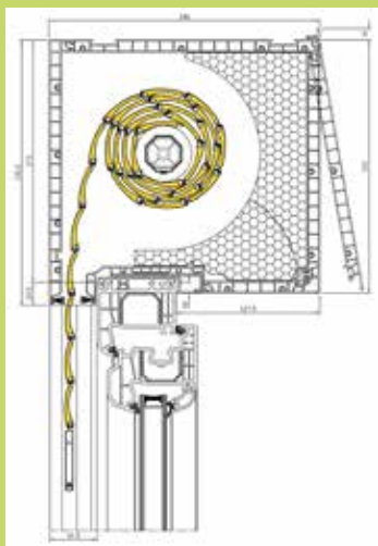
Snitt av rullgardinrulle.
